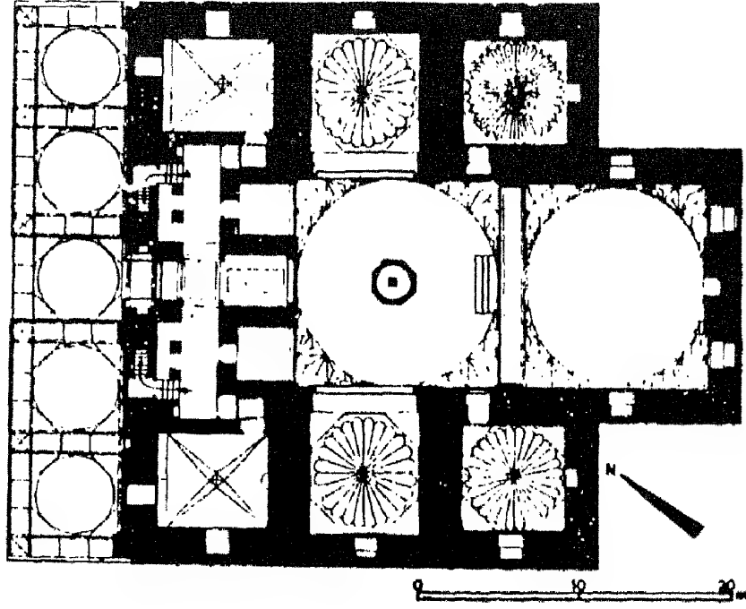
الشكل ٢٢-١٢ خطة جامع يشيل > بنية الوحدات المقنّبة < بورصة، تركيا ١٤١٢-١٤١٩ م.
